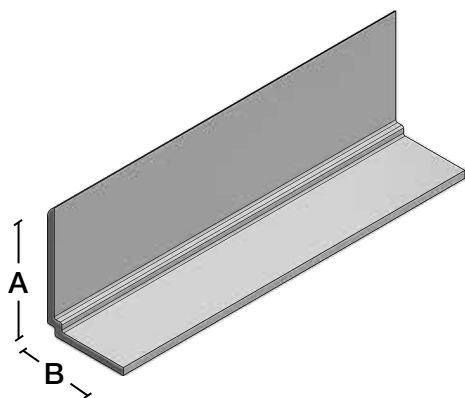
**Vista marco perimetral
