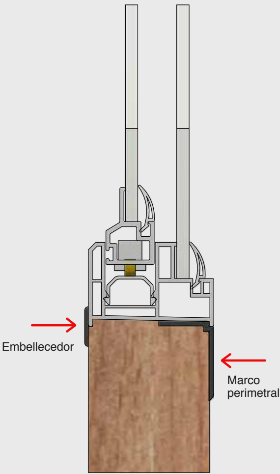
Vista embellecedor / marco perimetral
